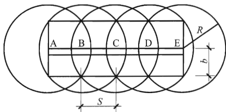
图 6 同层消火栓的布置示意图
